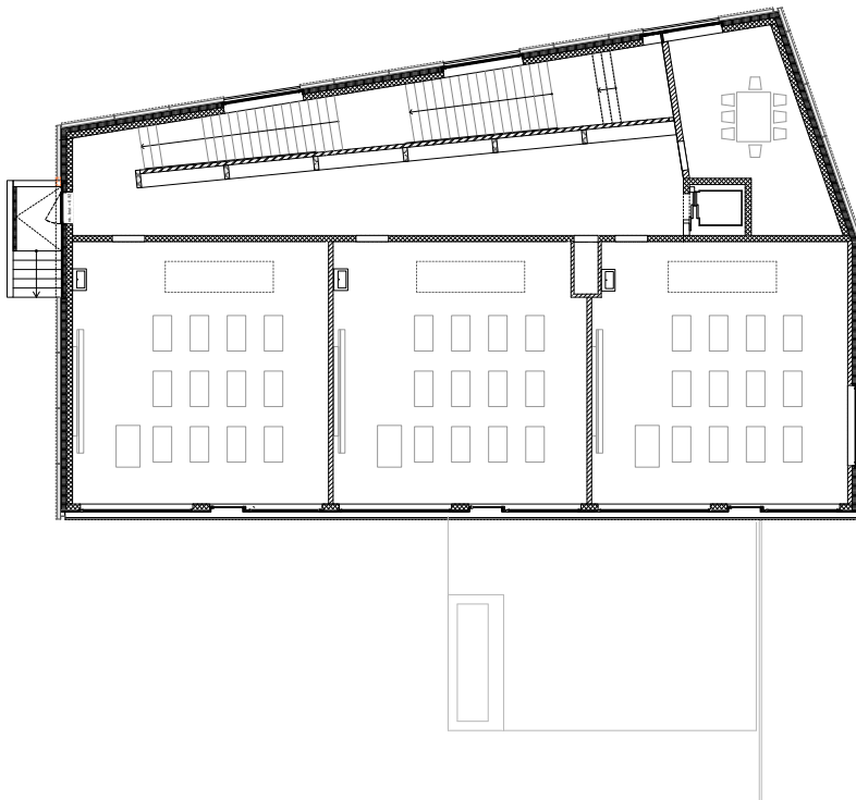
Plan +2
