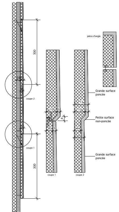
Coupe détail
