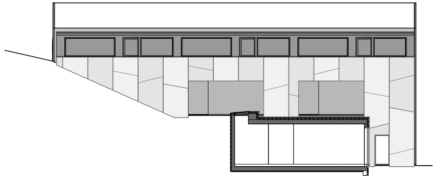
Elevation Sud
