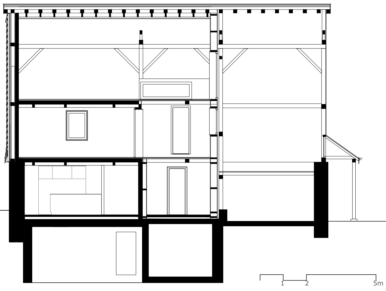
COUPE LONGITUDINALE
