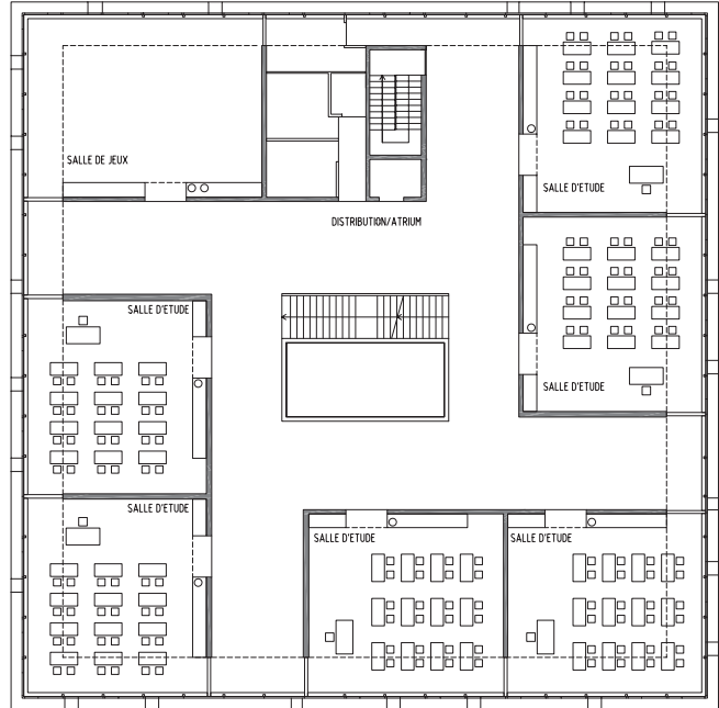
Plan d'étage type de l'école
