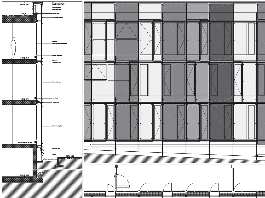
Plan, coupe et élévation de la façade double peau
