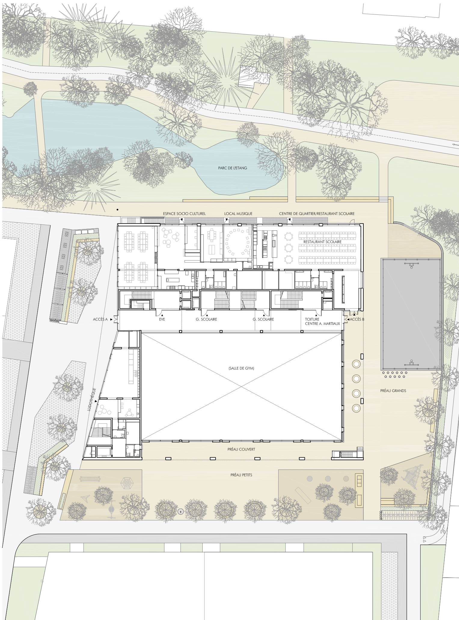
PLAN RDC+AMÉNAGEMENT EXTERIEUR
