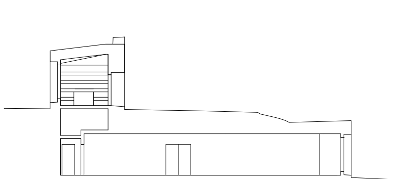
coupe longitudinale
