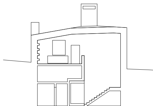
coupe transversale
