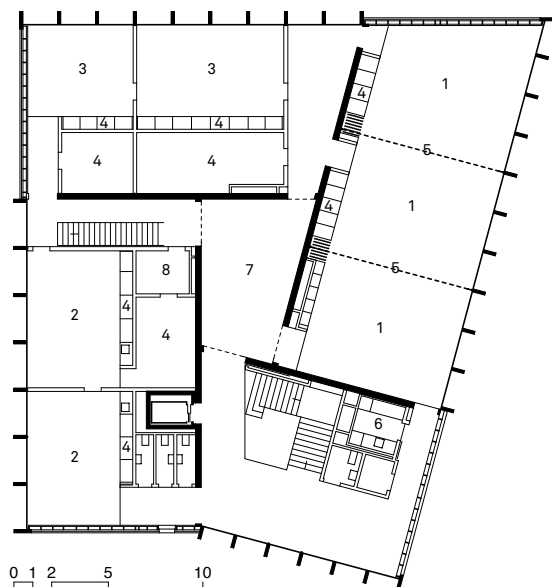
1er étage
