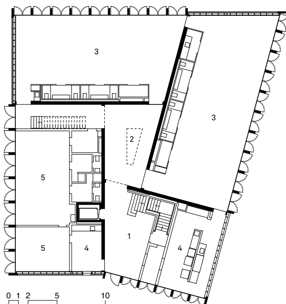
Rez-de-chaussée
